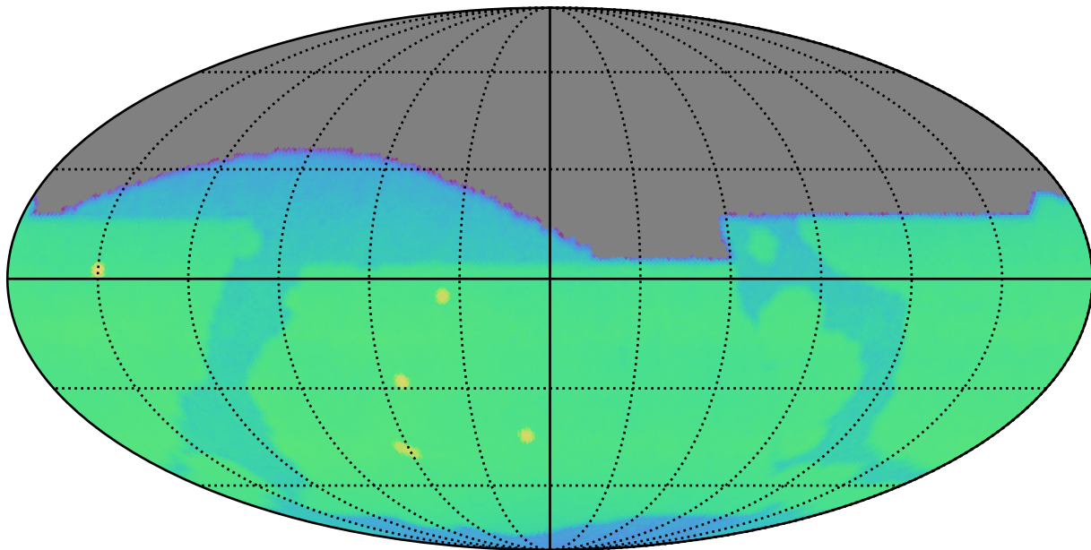
no_long_daily_v3.4_10yrs i: CoaddM5
