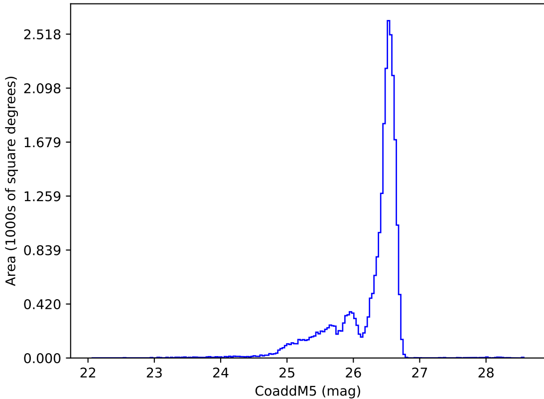
no_long_daily_v3.4_10yrs i: CoaddM5
