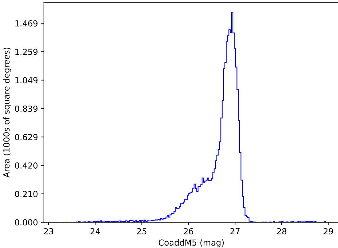
no_long_daily_v3.4_10yrs g: CoaddM5
