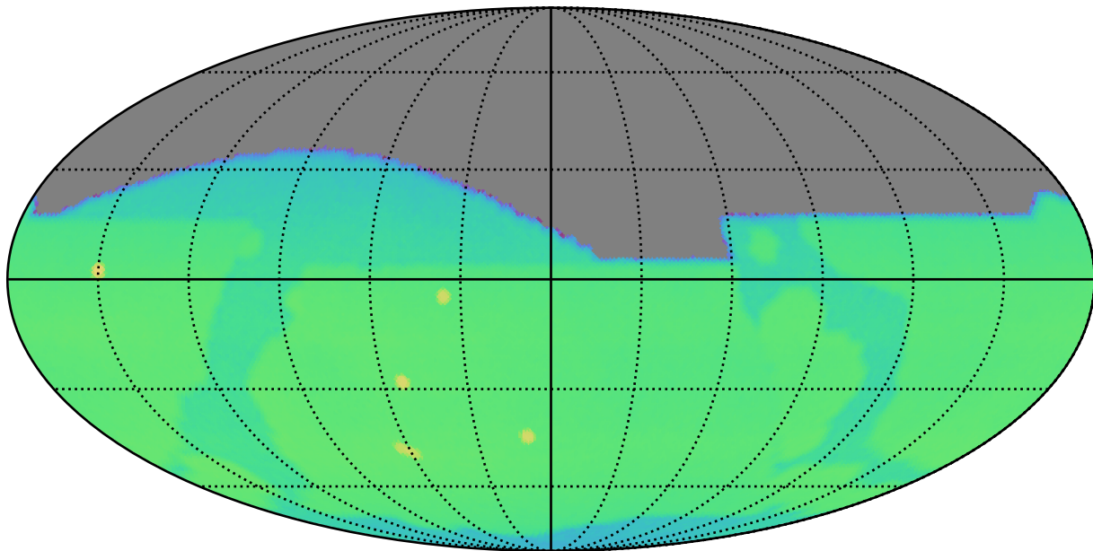
no_long_daily_v3.4_10yrs : CoaddM5
