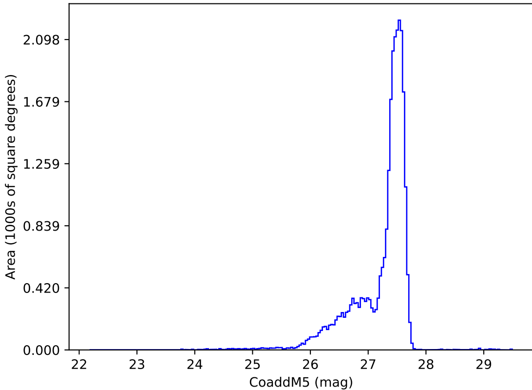
no_long_daily_v3.4_10yrs : CoaddM5
