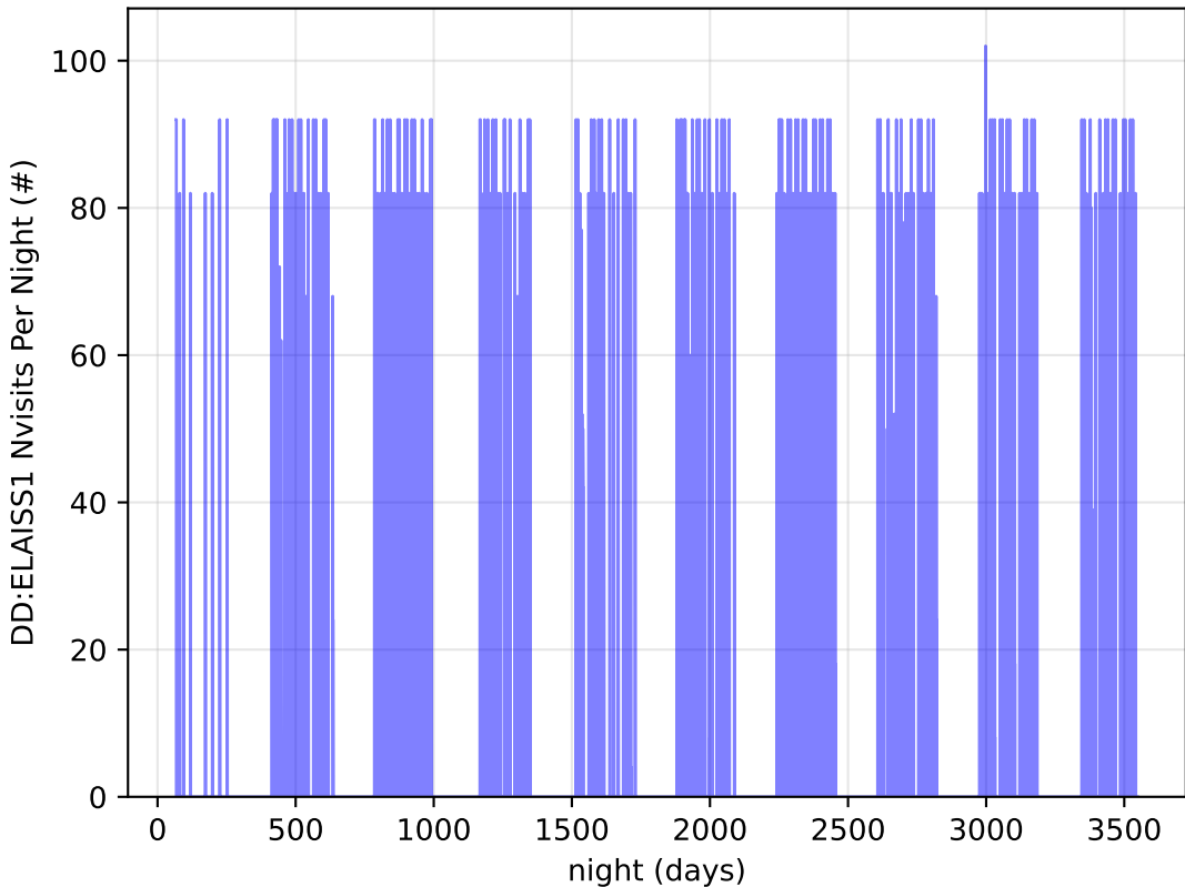
no_long_daily_v3.4_10yrs all bands: DD:ELAISS1 Nvisits Per Night
