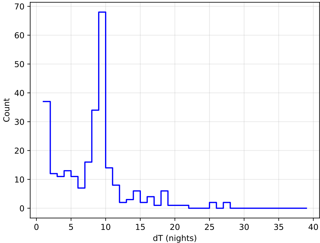
no_long_daily_v3.4_10yrs all bands: DD:ELAISS1 Delta Nights Histogram
