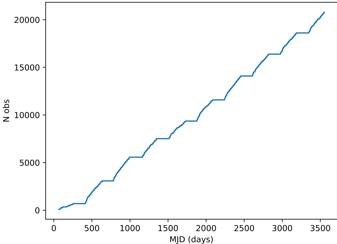
no_long_daily_v3.4_10yrs all bands: DD:ELAISS1 Cumulative NVisits
