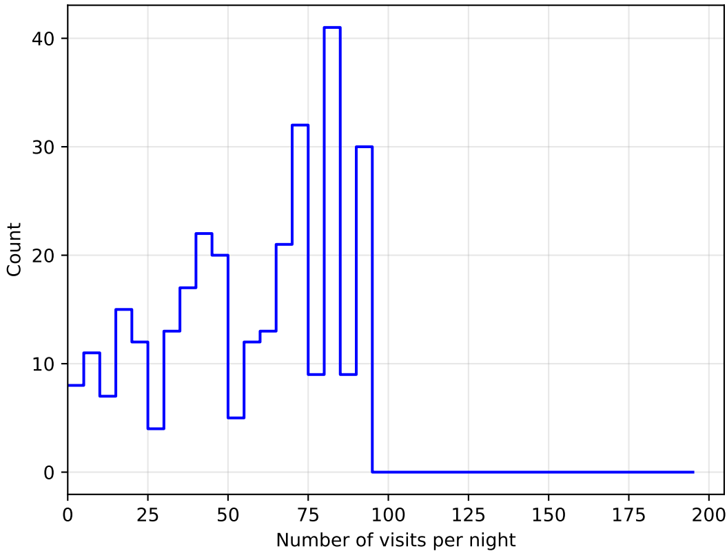
no_long_daily_v3.4_10yrs all bands: DD:EDFS NVisitsPerNight
