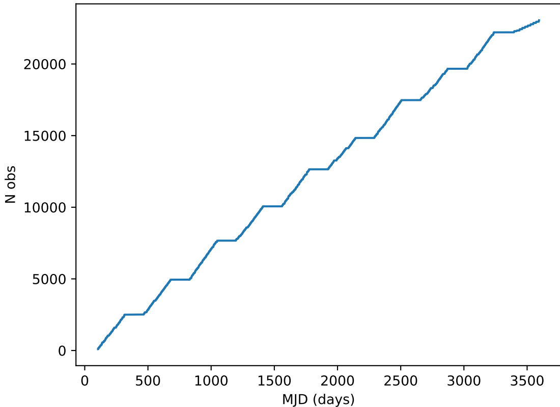
no_long_daily_v3.4_10yrs all bands: DD:EDFS Cumulative NVisits
