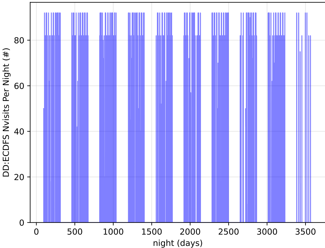
no_long_daily_v3.4_10yrs all bands: DD:ECDFS Nvisits Per Night
