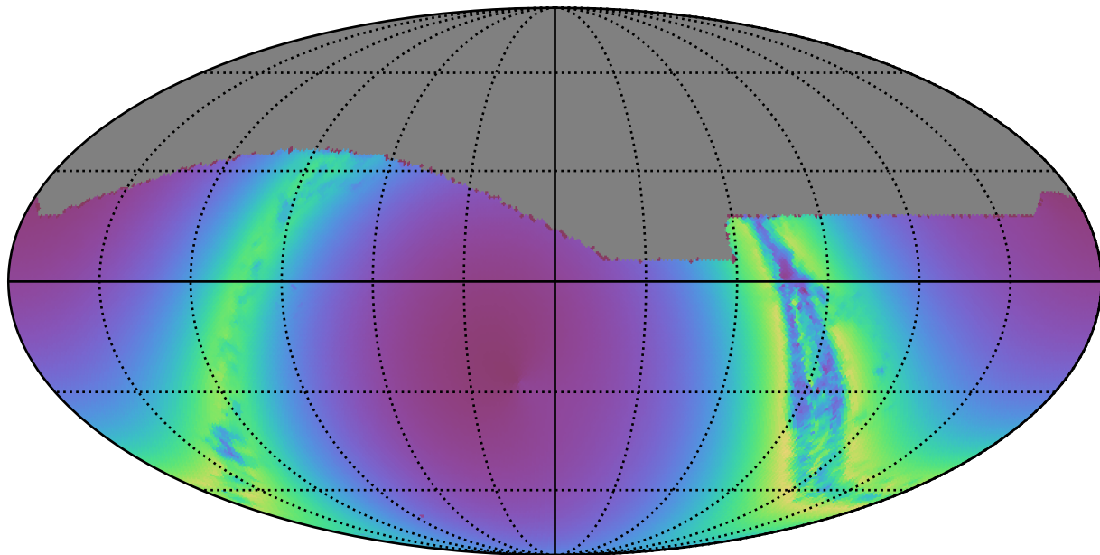
no_high_blob_v3.3_10yrs : young_stars
