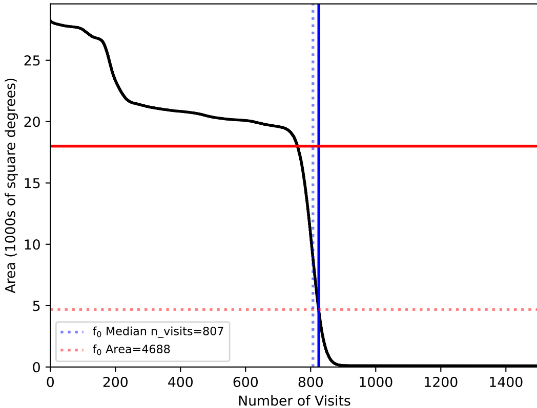
no_high_blob_v3.3_10yrs : f0
