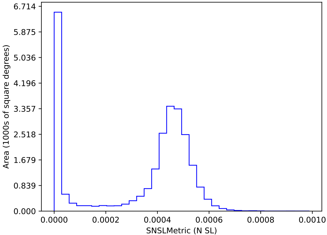
no_high_blob_v3.3_10yrs : SNSLMetric
