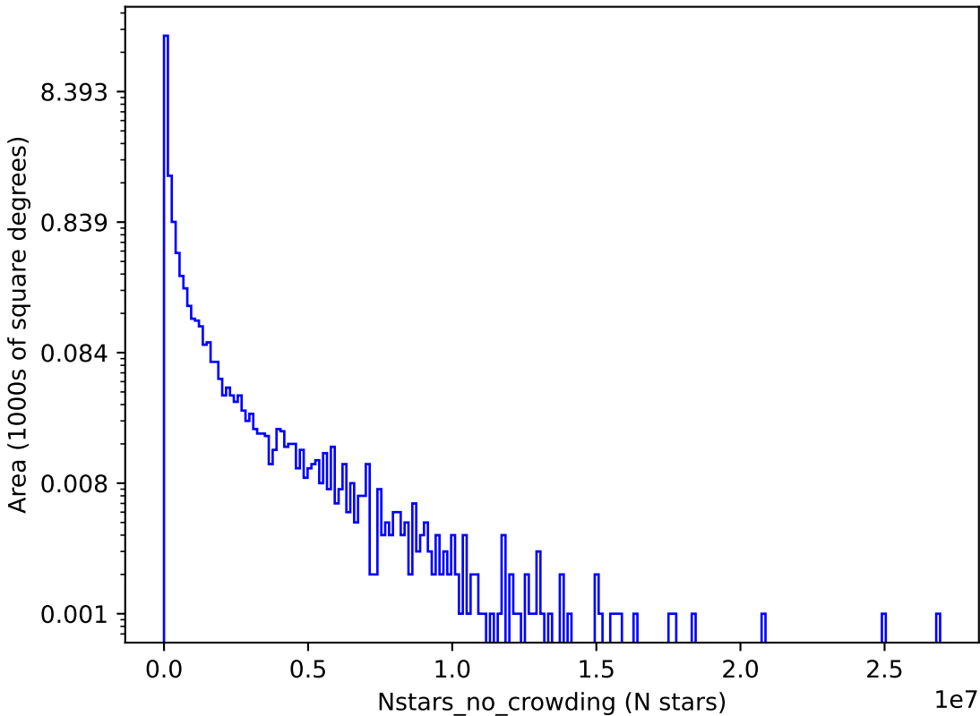
no_high_blob_v3.3_10yrs z: Nstars_no_crowding
