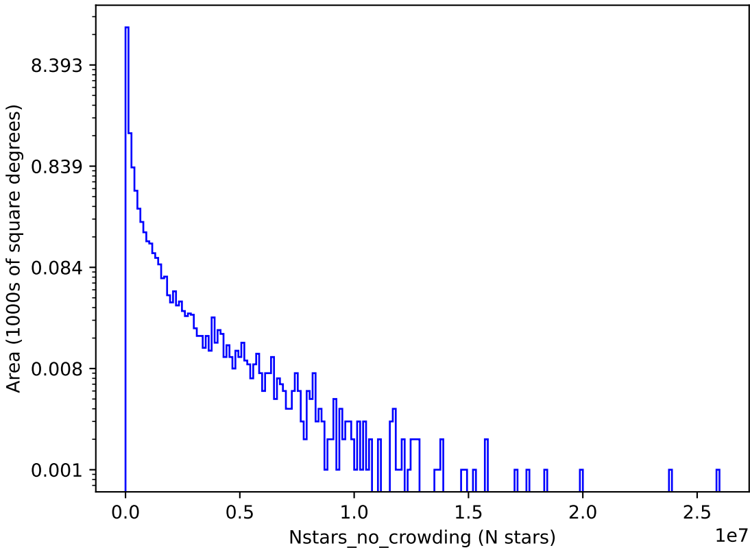
no_high_blob_v3.3_10yrs y: Nstars_no_crowding
