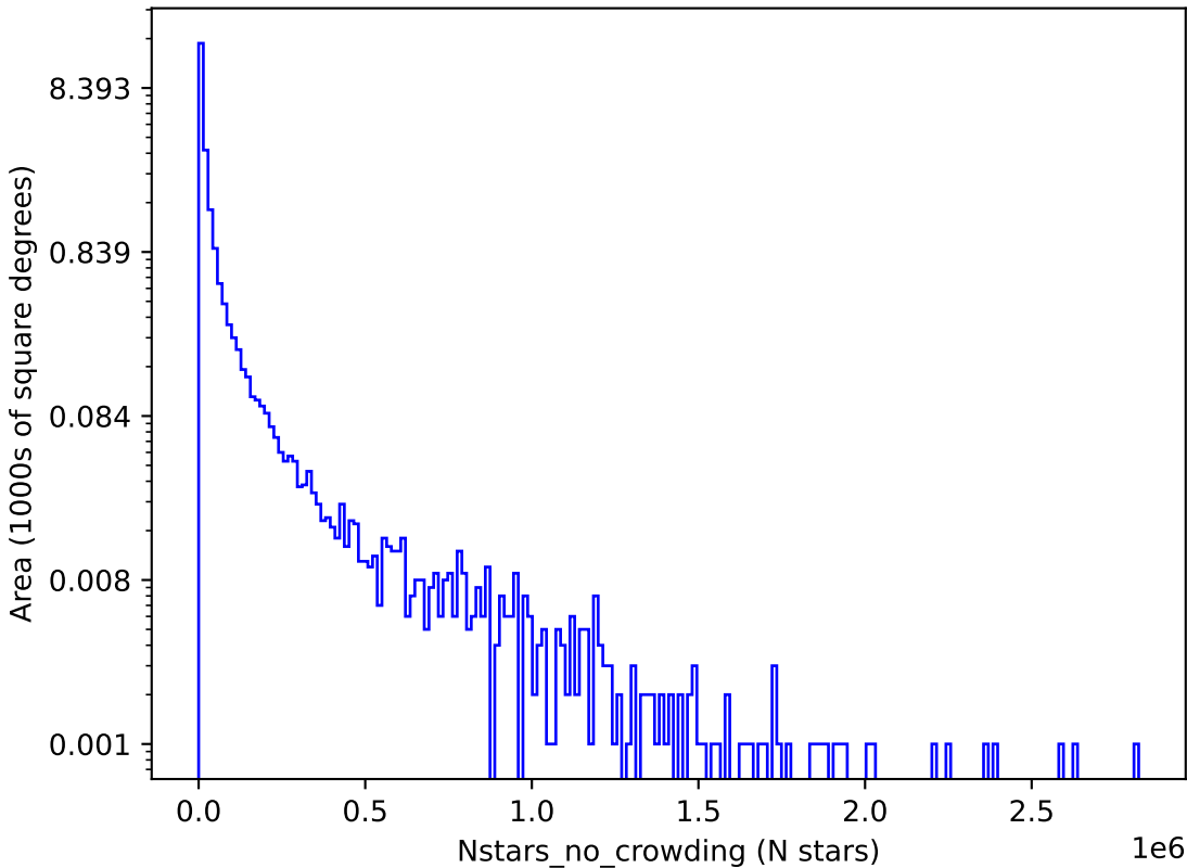
no_high_blob_v3.3_10yrs u: Nstars_no_crowding
