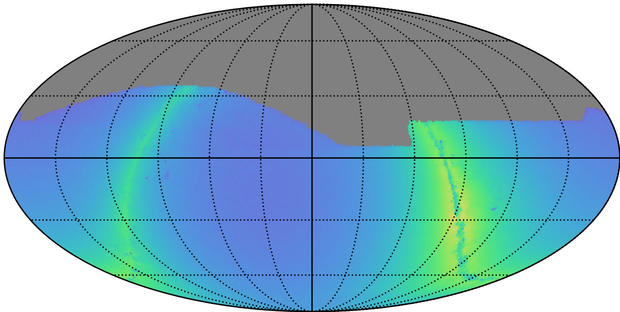
no_high_blob_v3.3_10yrs i: Nstars_no_crowding
