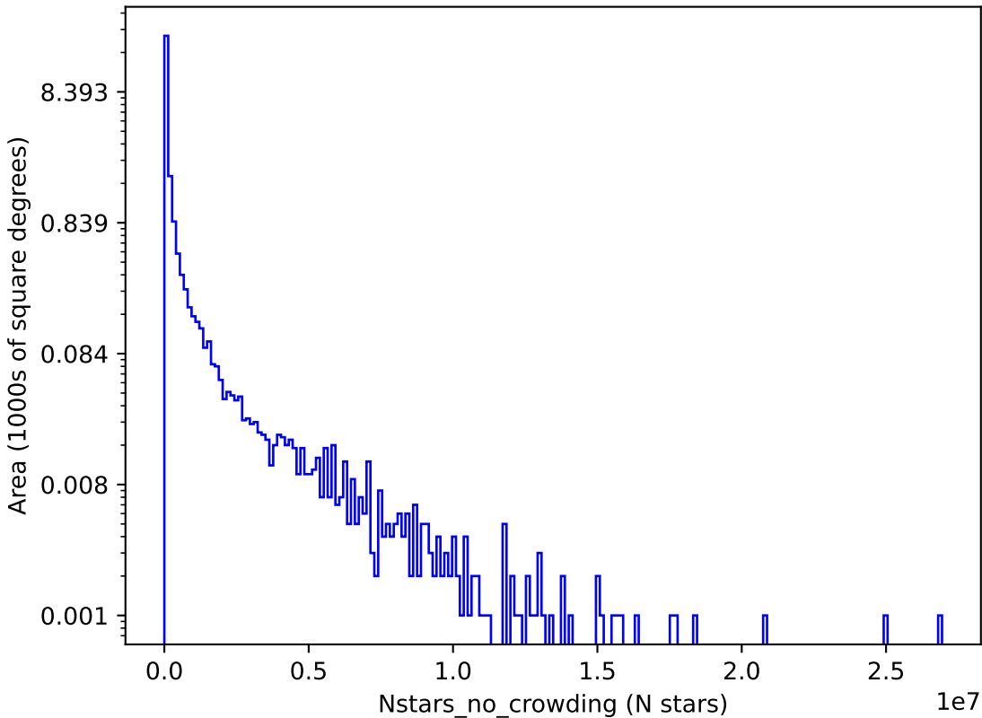
no_high_blob_v3.3_10yrs i: Nstars_no_crowding
