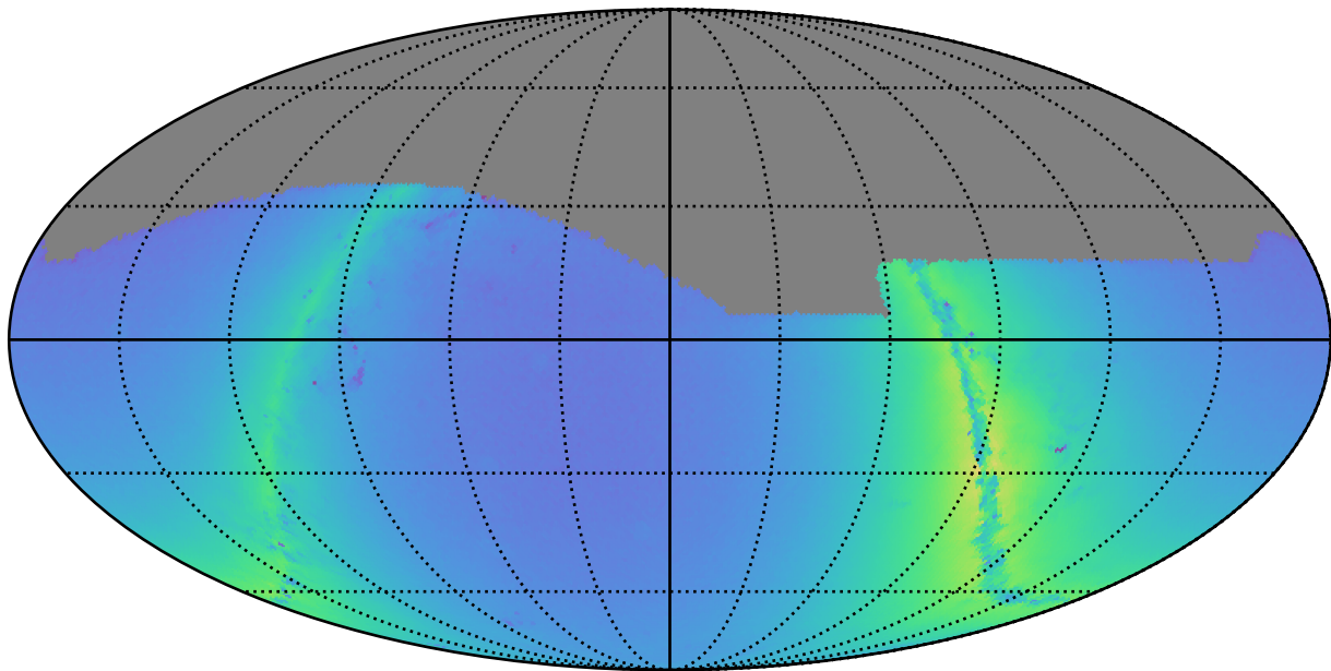
no_high_blob_v3.3_10yrs g: Nstars_no_crowding
