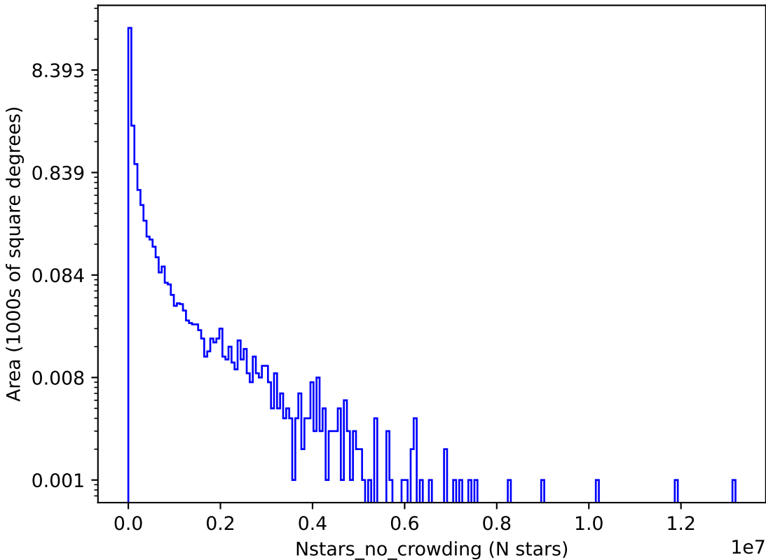
no_high_blob_v3.3_10yrs g: Nstars_no_crowding
