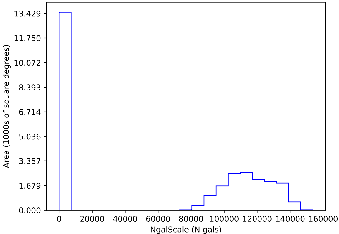
no_high_blob_v3.3_10yrs i: NgalScale
