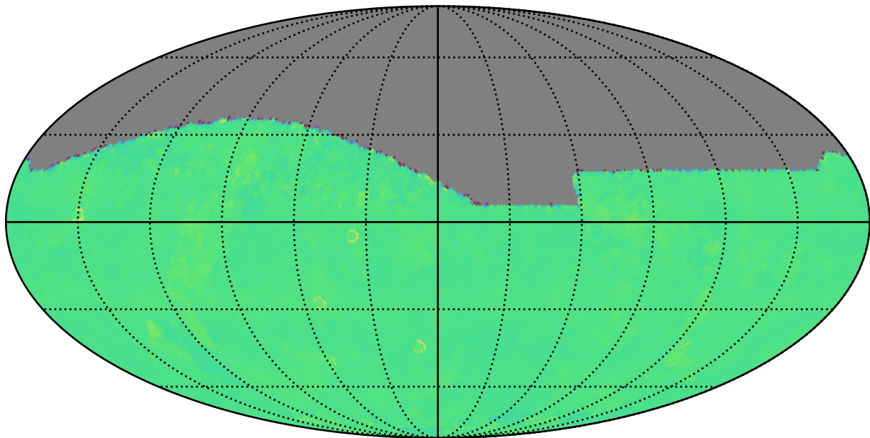
no_high_blob_v3.3_10yrs z: Kuiper rotTelPos
