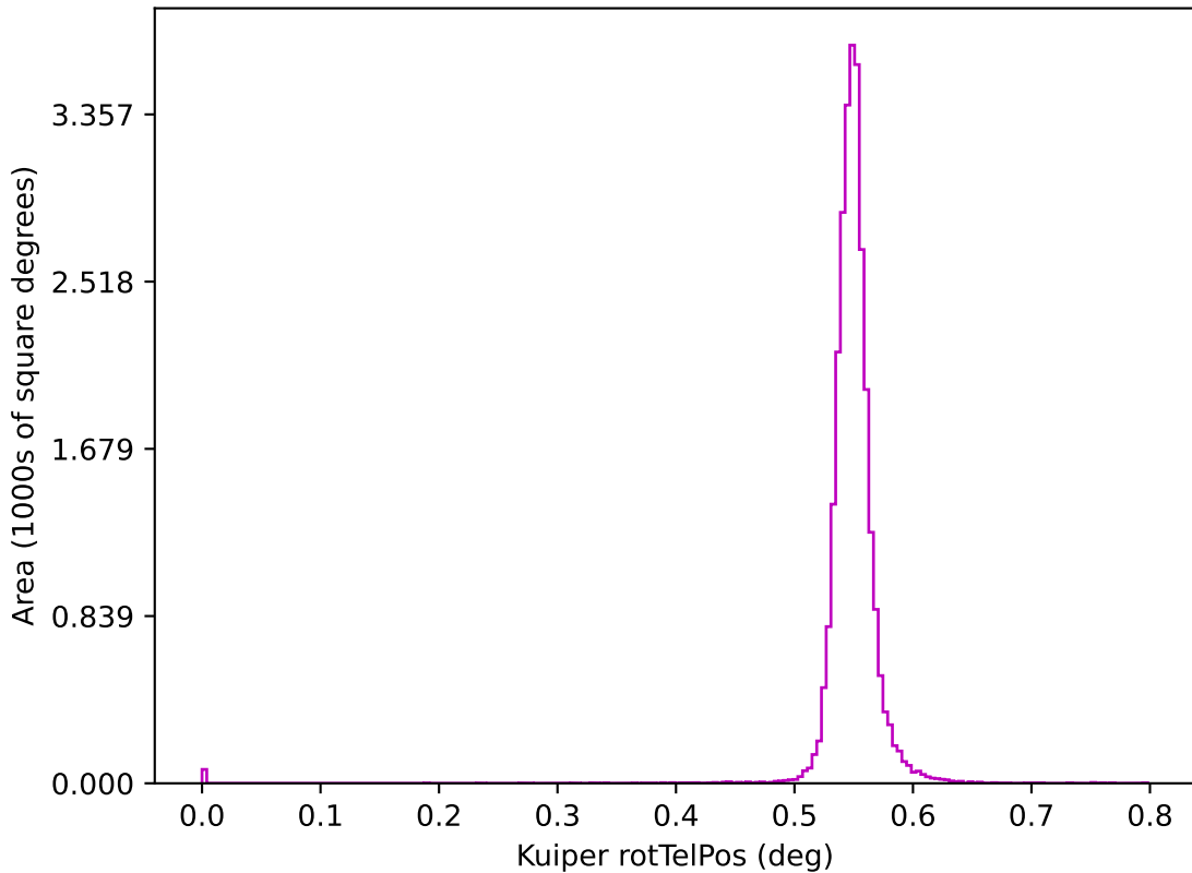
no_high_blob_v3.3_10yrs z: Kuiper rotTelPos
