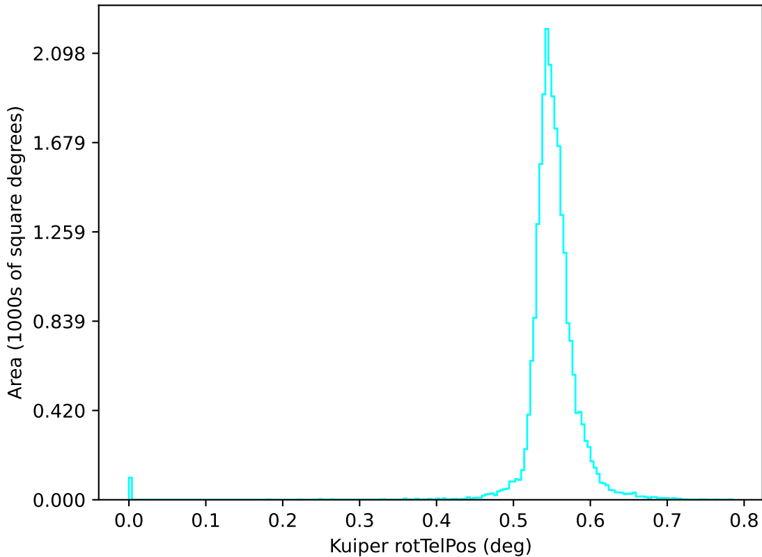
no_high_blob_v3.3_10yrs u: Kuiper rotTelPos
