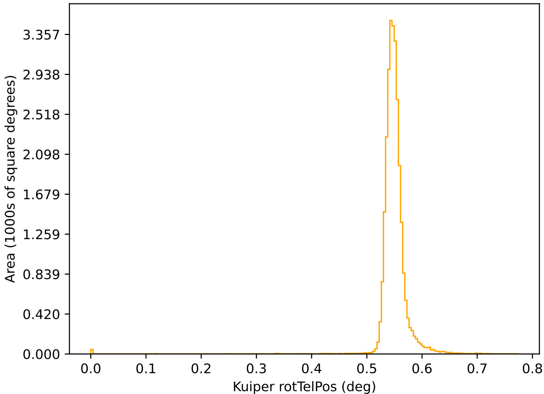
no_high_blob_v3.3_10yrs r: Kuiper rotTelPos
