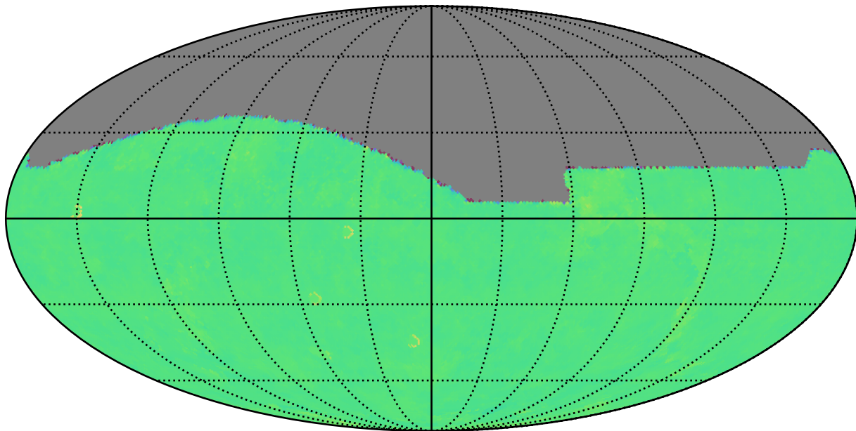
no_high_blob_v3.3_10yrs i: Kuiper rotTelPos
