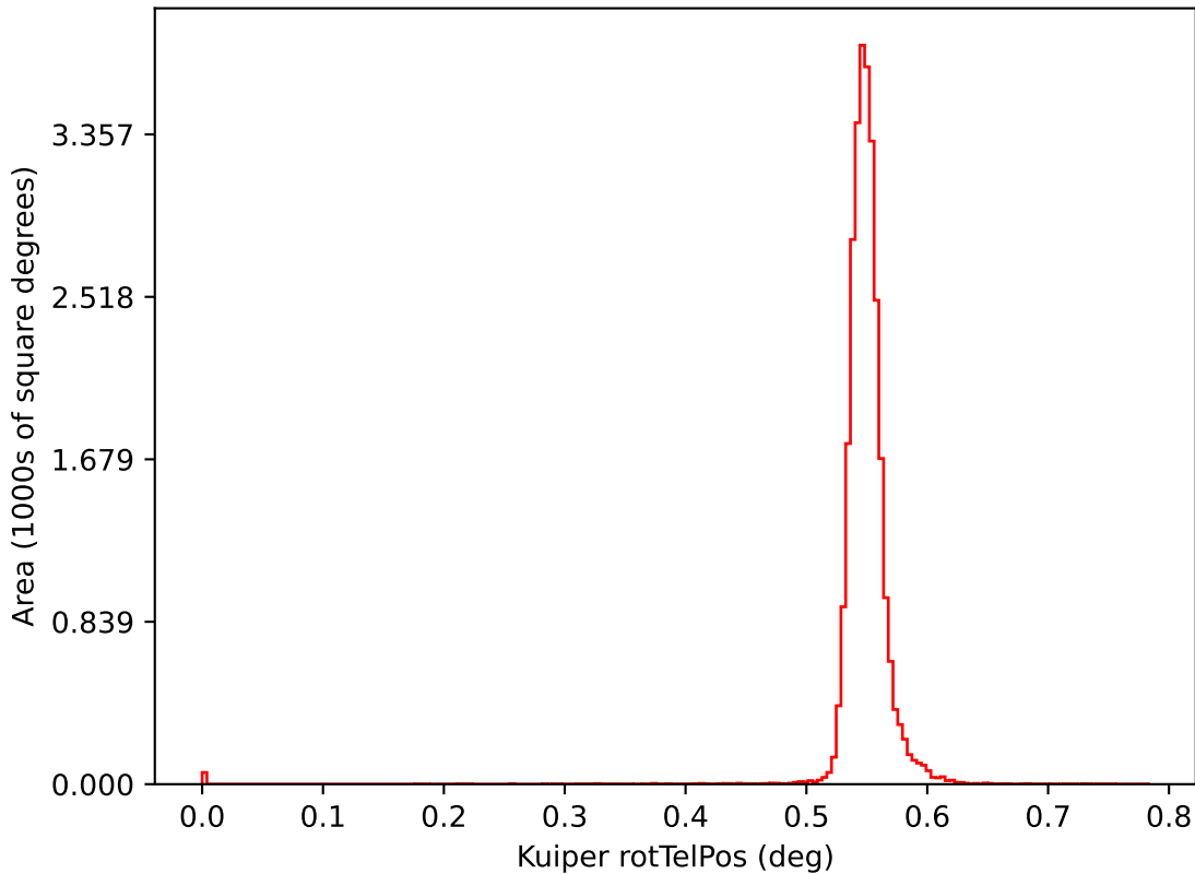
no_high_blob_v3.3_10yrs i: Kuiper rotTelPos
