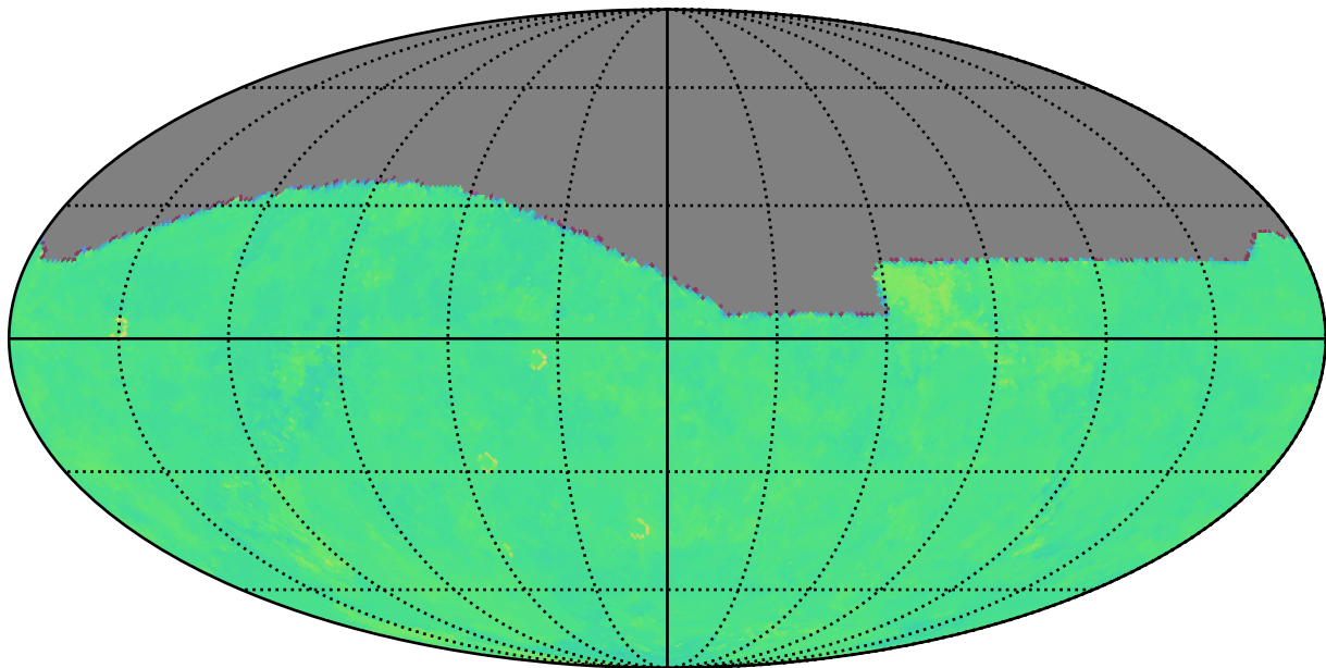
no_high_blob_v3.3_10yrs g: Kuiper rotTelPos
