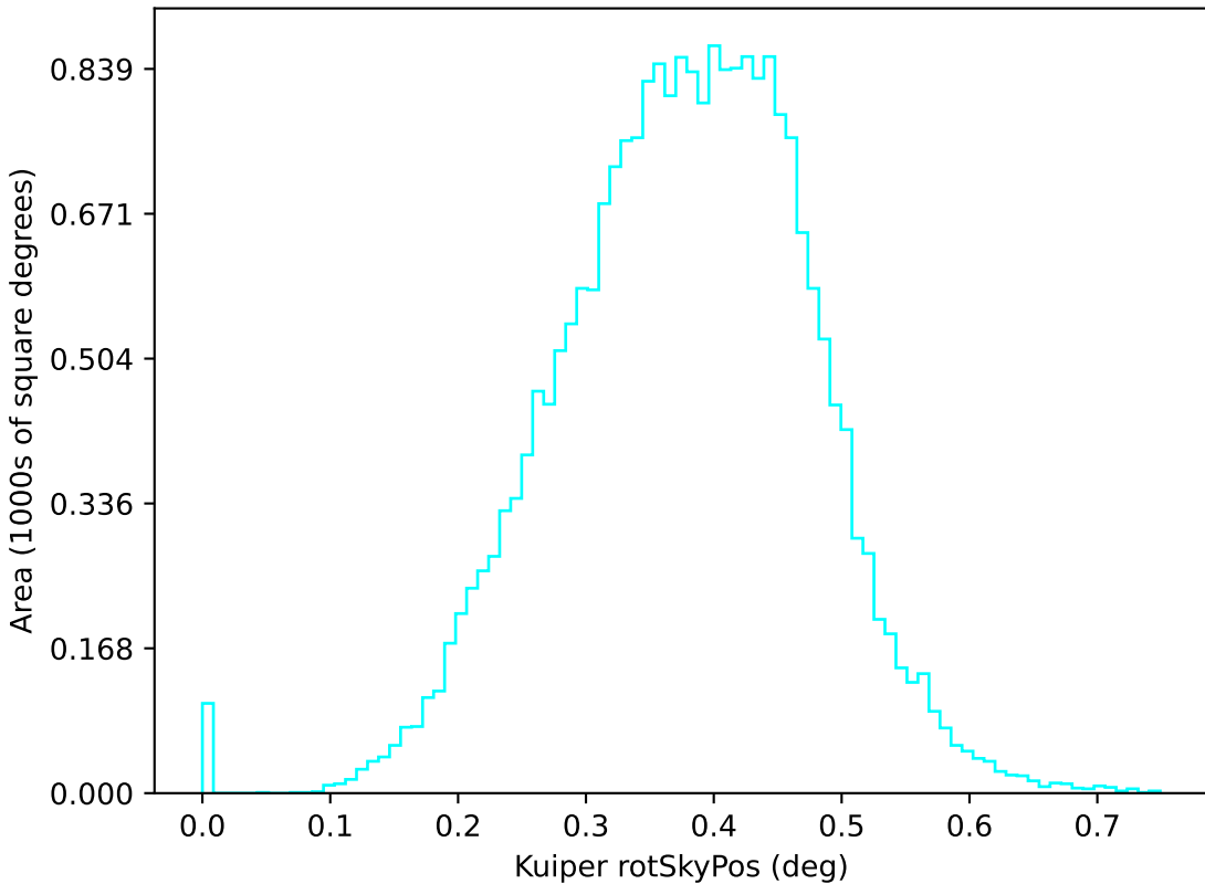
no_high_blob_v3.3_10yrs u: Kuiper rotSkyPos
