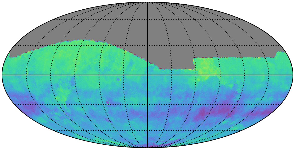
no_high_blob_v3.3_10yrs i: Kuiper rotSkyPos
