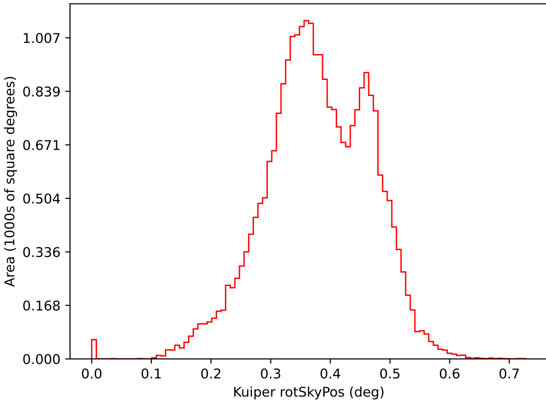
no_high_blob_v3.3_10yrs i: Kuiper rotSkyPos
