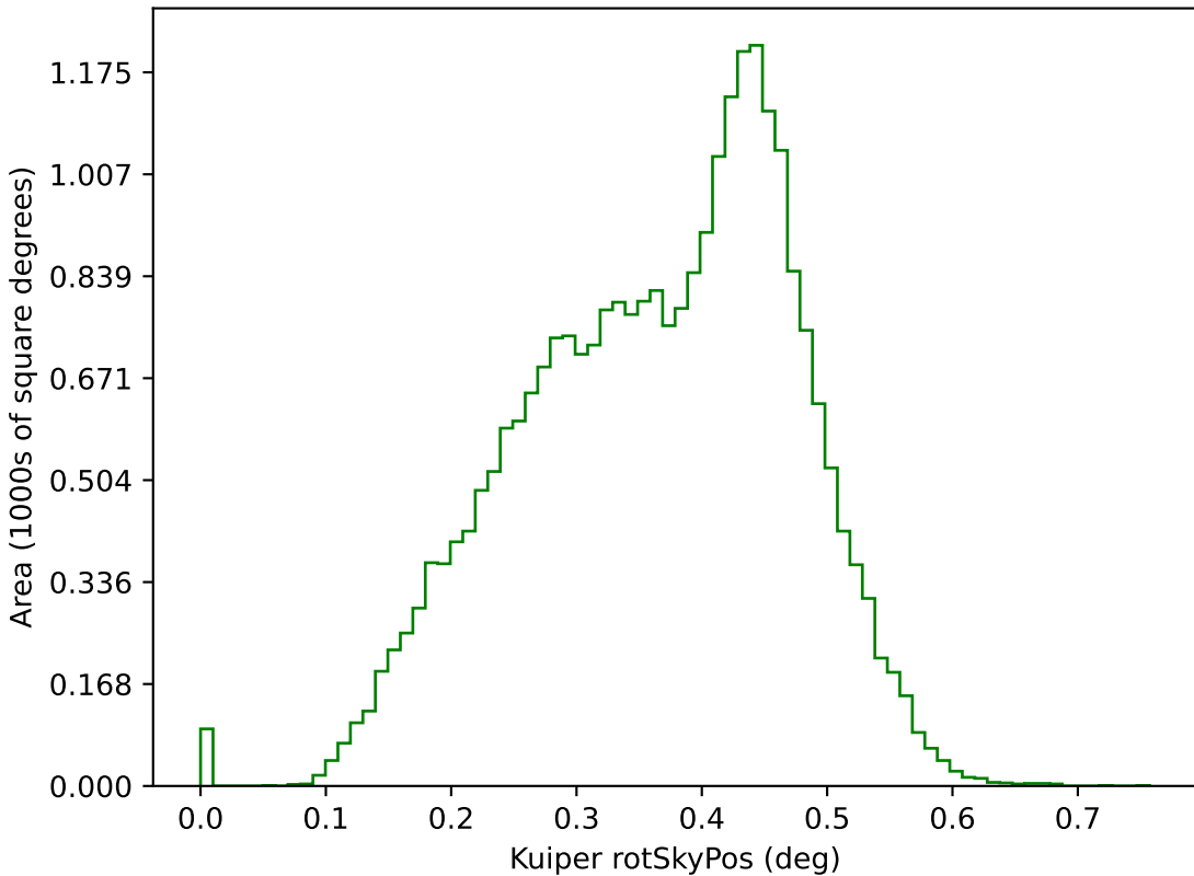
no_high_blob_v3.3_10yrs g: Kuiper rotSkyPos
