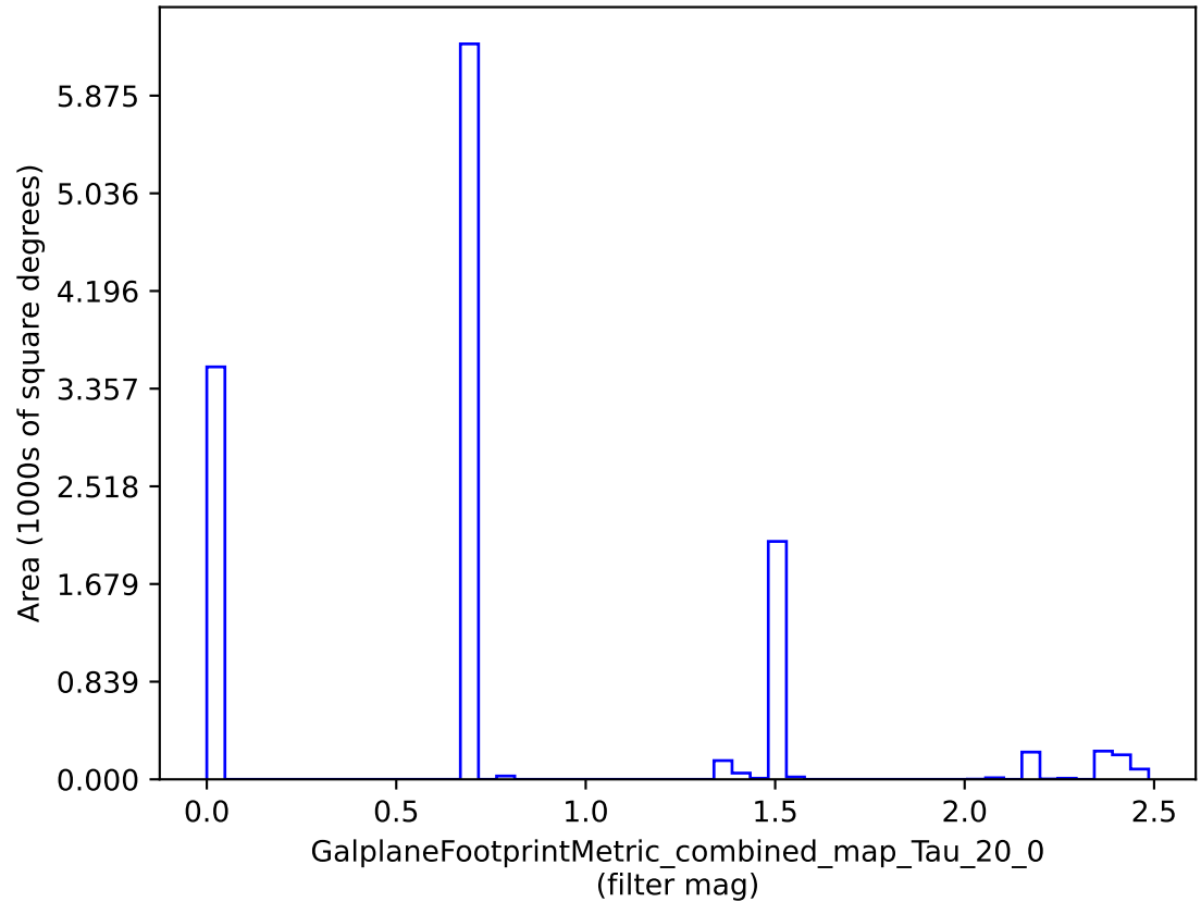
no_high_blob_v3.3_10yrs : GalplaneFootprintMetric_combined_map_Tau_20_0
