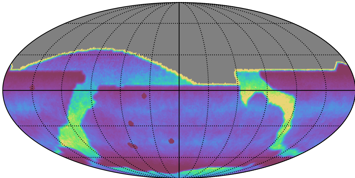
no_high_blob_v3.3_10yrs : DCRprecision
