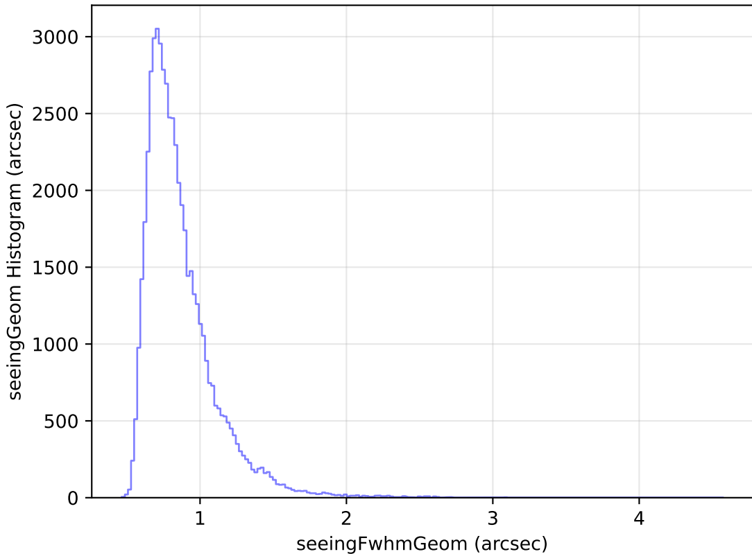
no_high_blob_v3.3_10yrs Yr 1 i band: seeingGeom Histogram
