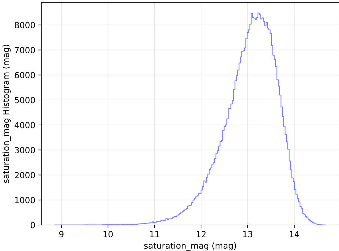
no_high_blob_v3.3_10yrs WFD y band: saturation_mag Histogram
