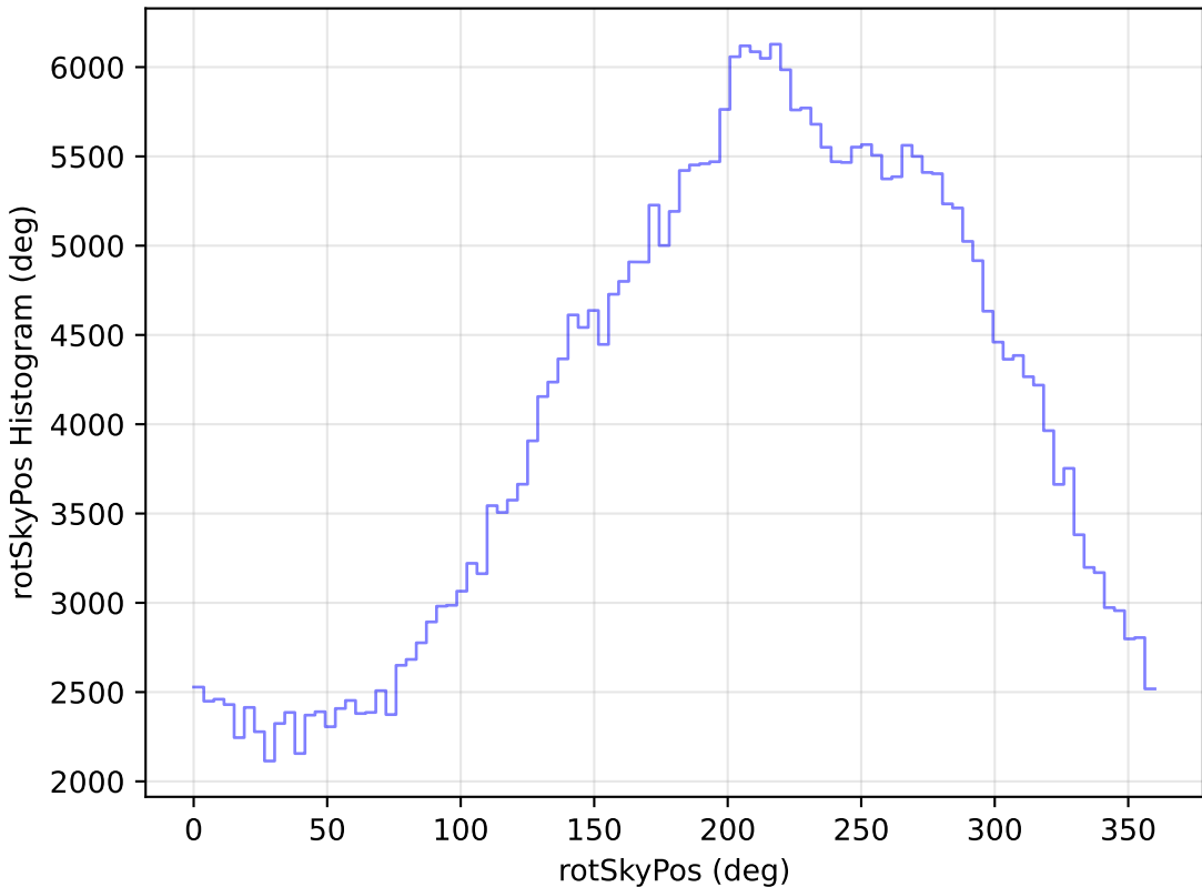
no_high_blob_v3.3_10yrs WFD y band: rotSkyPos Histogram
