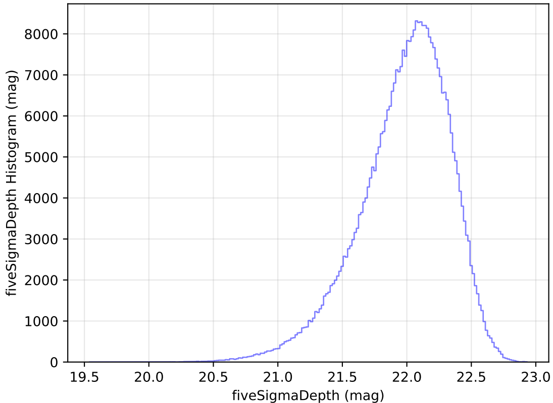
no_high_blob_v3.3_10yrs WFD y band: fiveSigmaDepth Histogram
