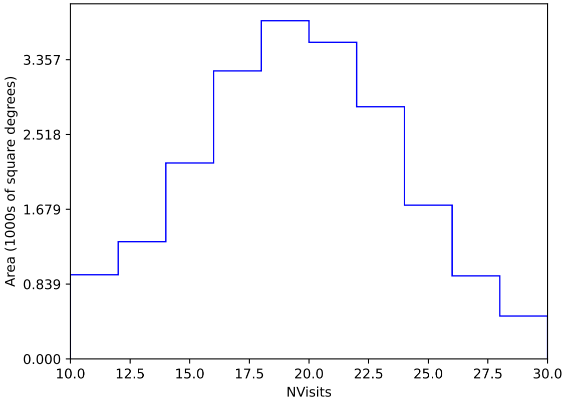
no_high_blob_v3.3_10yrs Yr 1 y band: NVisits
