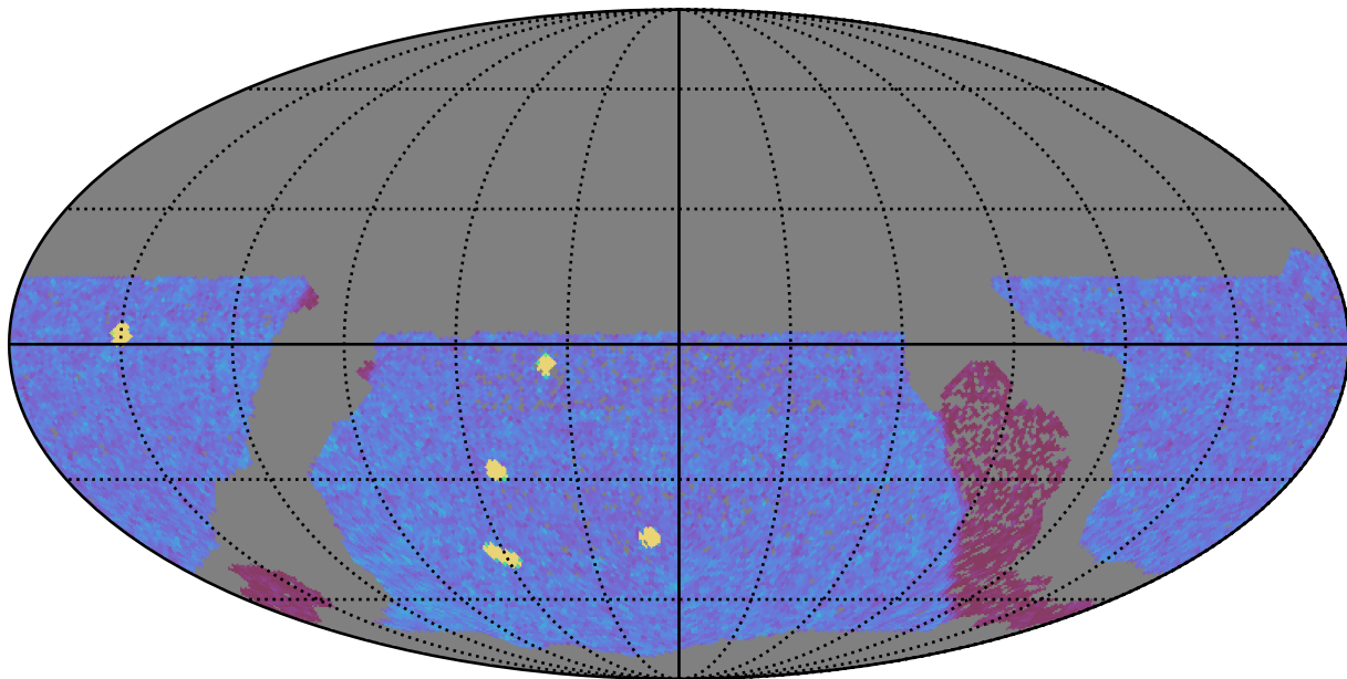
no_high_blob_v3.3_10yrs WFD y band: NVisits
