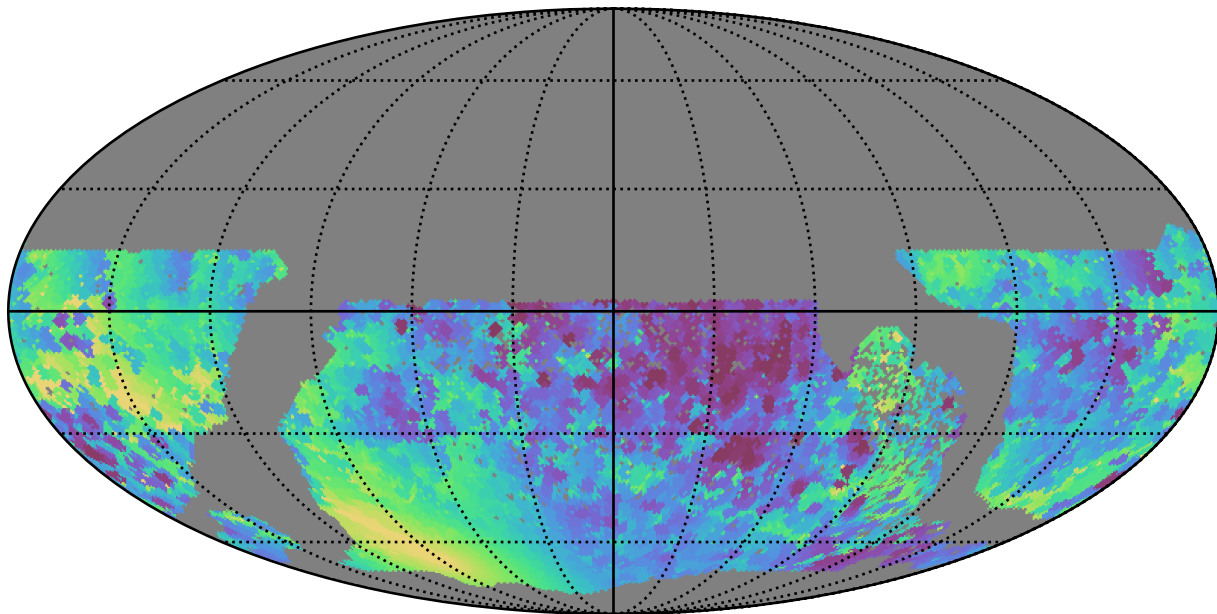
no_high_blob_v3.3_10yrs WFD y band: Min solarElong
