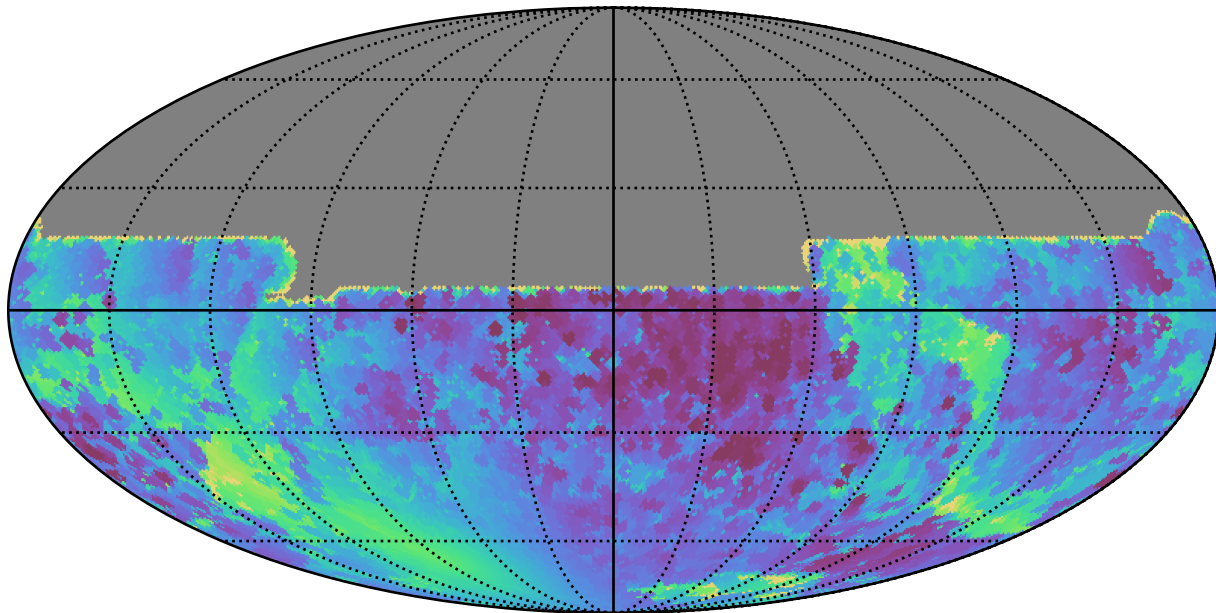
no_high_blob_v3.3_10yrs All sky y band: Min solarElong
