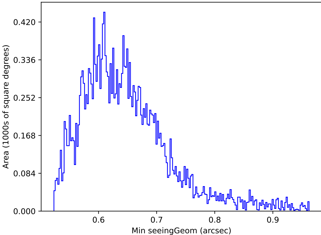
no_high_blob_v3.3_10yrs Yr 1 y band: Min seeingGeom
