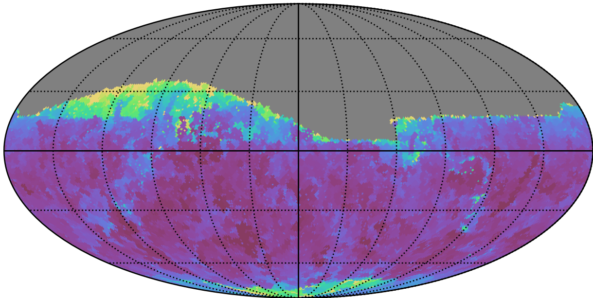
no_high_blob_v3.3_10yrs Yr 1 i band: Min seeingGeom
