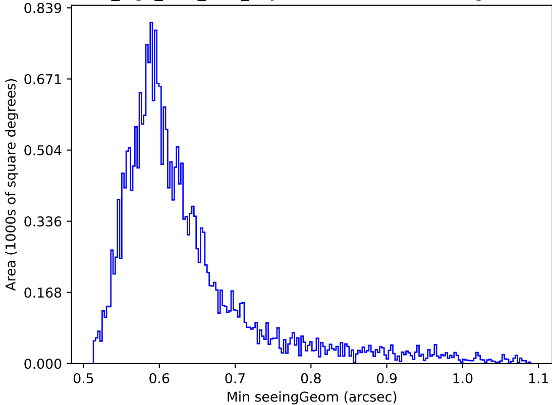
no_high_blob_v3.3_10yrs Yr 1 i band: Min seeingGeom
