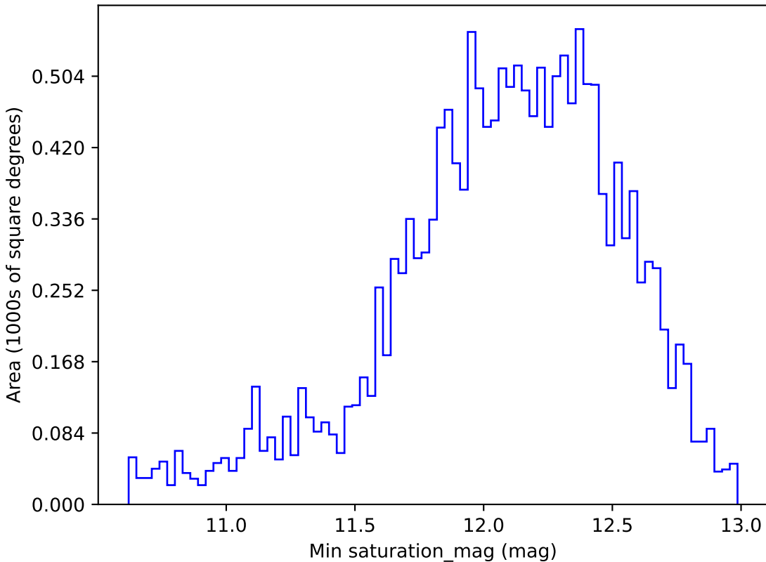
no_high_blob_v3.3_10yrs WFD z band: Min saturation_mag
