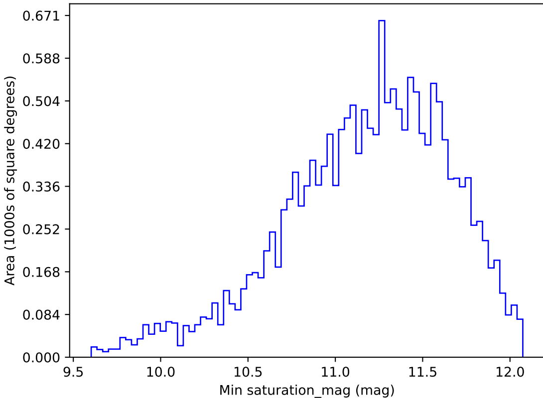
no_high_blob_v3.3_10yrs WFD y band: Min saturation_mag
