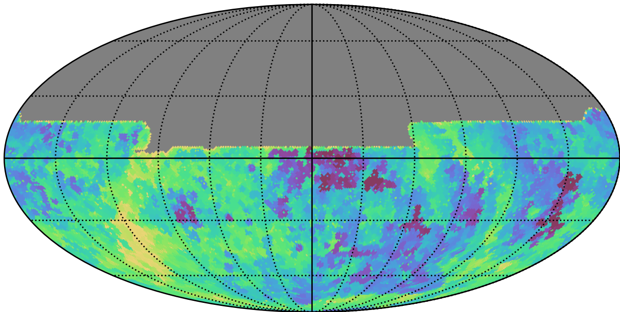
no_high_blob_v3.3_10yrs All sky y band: Min saturation_mag
