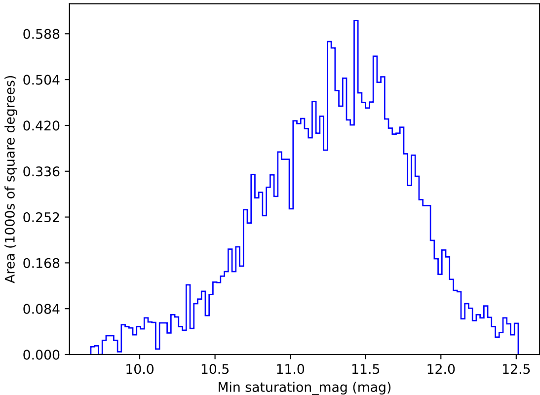
no_high_blob_v3.3_10yrs All sky y band: Min saturation_mag
